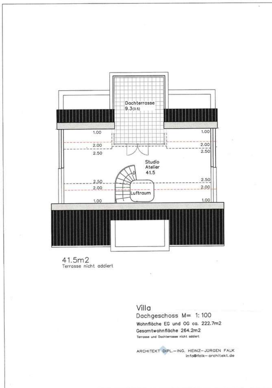
Grundriss DG
