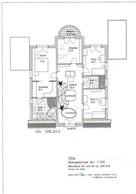
Grundriss OG
