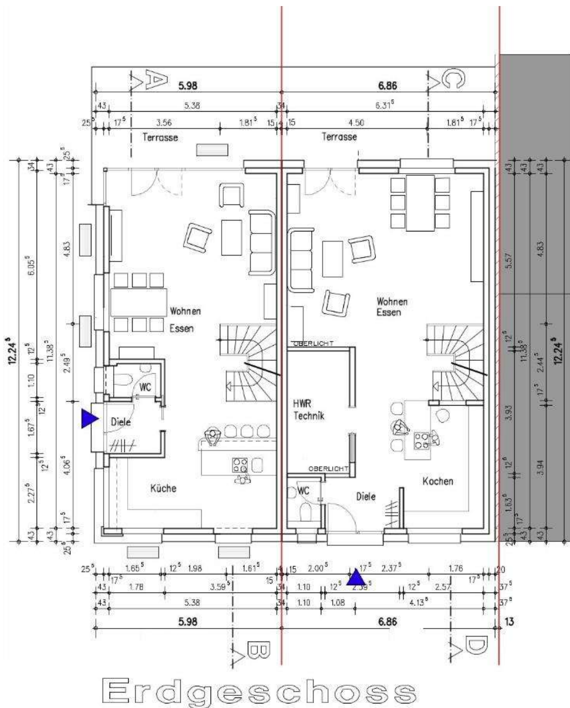
Grundriss EG Beispiel
