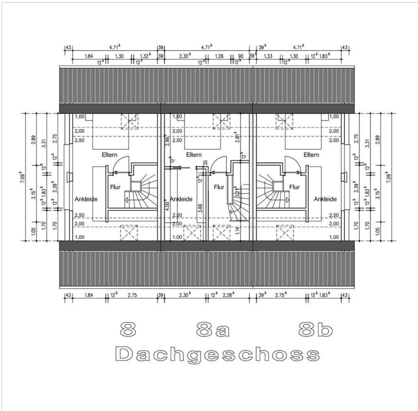
Grundriss DG
