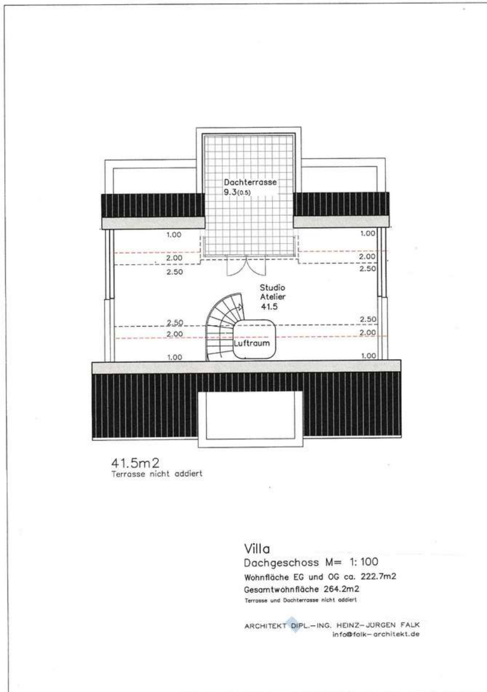
Grundriss DG
