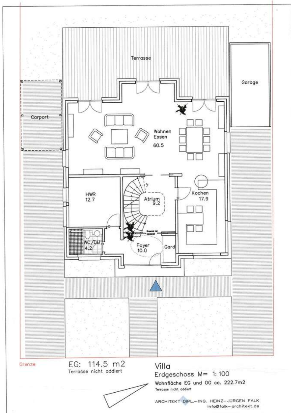
Grundriss EG
